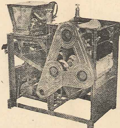
市原式落花生脱皮機B型
